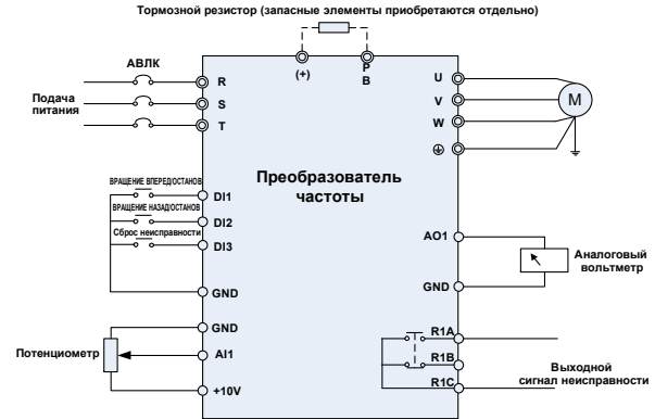
Рисунок 6. Схема подключения
