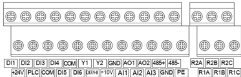
Рис. 3-15. Клеммы цепи управления
