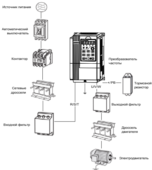
Рис. 3-9. Стандартная конфигурация периферийных устройств
