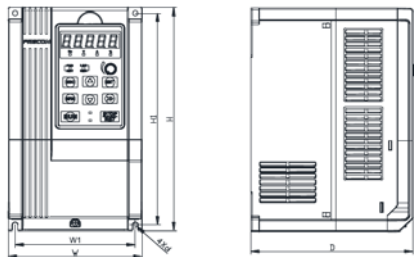
Рис. 2-5. Схема настенного монтажа ПЧ мощностью 4~22 кВт
