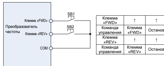
Рисунок 6-12. Схема импульсного управления остановом
