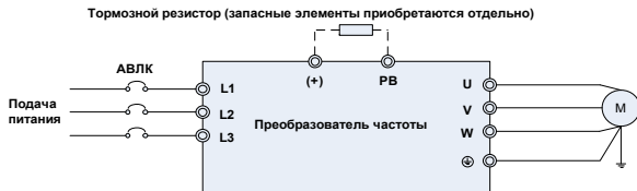
Рисунок 2. Схема подключения силовых цепей
