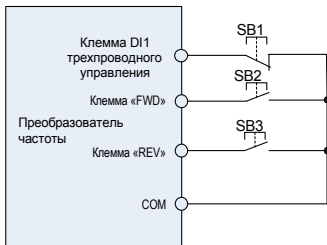
Рисунок 6-10. Настройки режима трехпроводного управления 1
