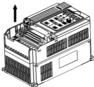
Рисунок В-4. Снятие модуля выгрузки и загрузки
