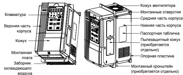
Рис. 2-3-б. Схематическое изображение ПЧ мощностью 4~22 кВт
