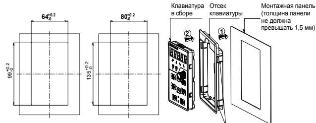
Рис. 2-11. Схема установки внешней клавиатуры ПЧ мощностью 0,75–630 кВт с габаритными чертежами
