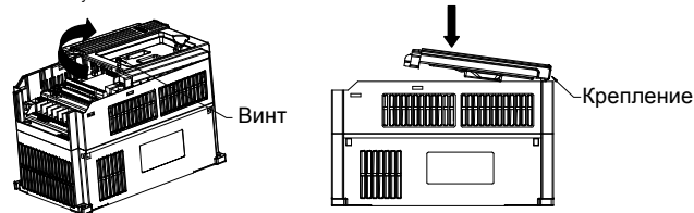
Рис. 3-7(ф). Демонтаж и монтаж кожуха
