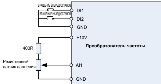
Рисунок 5. Схема подключения цепей управления
