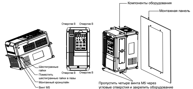
Рис. 3-6. Настенный монтаж ПЧ мощностью 4~22 кВт
