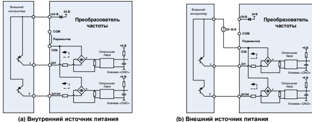
Рис. 3-19. PNP-подключение внешнего источника питания с открытым коллектором
