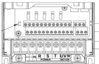
Рис. 3-11. Схема силовых клемм ПЧ мощностью 4~5,5 кВт
