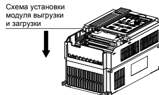
Рисунок В-2. Установка модуля выгрузки и загрузки
