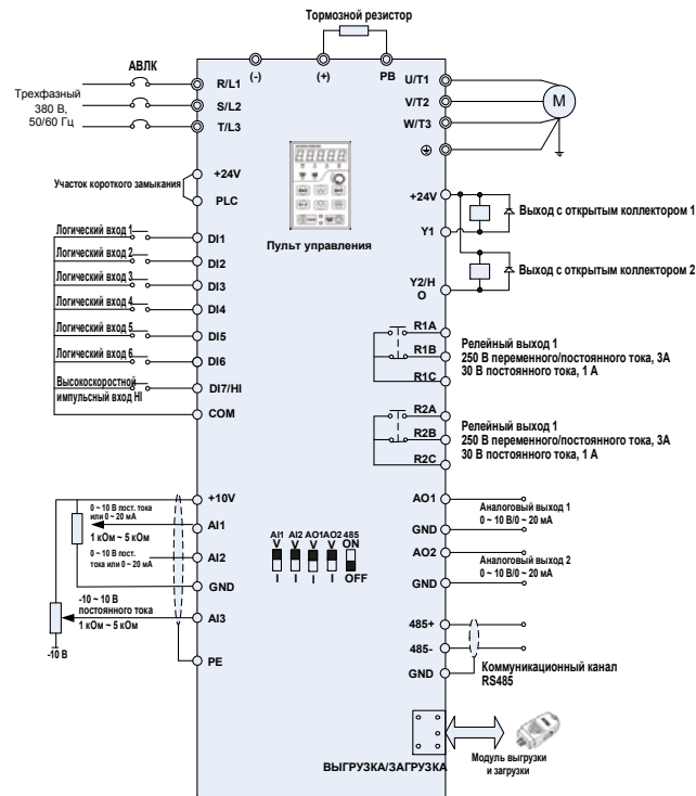
Рис.3-10 Стандартная схема подключения преобразователя частоты PM500A
