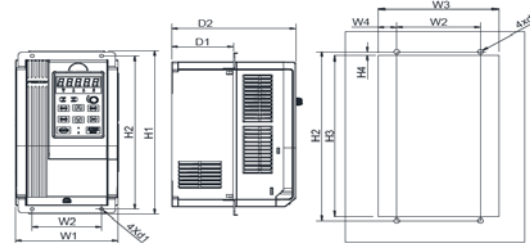
Рис. 2-7. Схема фланцевого монтажа ПЧ мощностью 4~22 кВт
