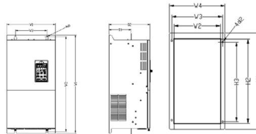
Рис. 2-8. Схема фланцевого монтажа ПЧ мощностью 30~90 кВт
