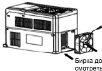
Рисунок 8-2 (а). Установка вентилятора
