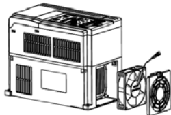
Рисунок 8-1 (б). Демонтаж вентилятора
