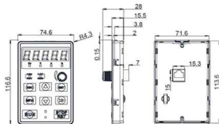
Рис. 2-9. Габаритный чертеж клавиатуры ПЧ мощностью 4,0–160 кВт
