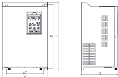
Рис. 2-6. Схема настенного монтажа ПЧ мощностью 30~160 кВт
