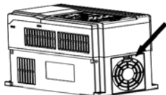
Рисунок 8-1 (а). Демонтаж кожуха вентилятора
