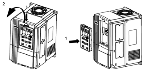
Рис. 3-7(а). Демонтаж клавиатуры
