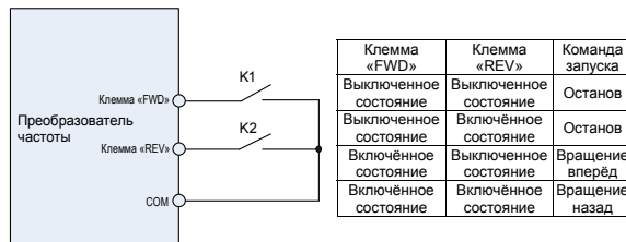
Рисунок 6-9. Настройки режима двухпроводного управления 2
