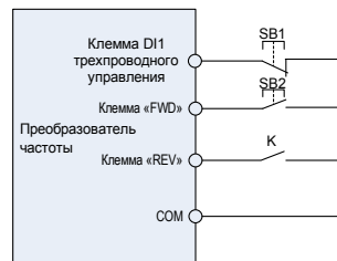
Рисунок 6-11. Настройки режима трехпроводного управления 2
