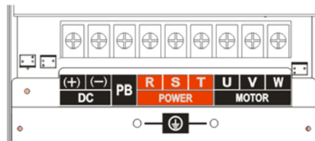
Рис. 3-13. Схема силовых клемм ПЧ мощностью 30~37 кВт
