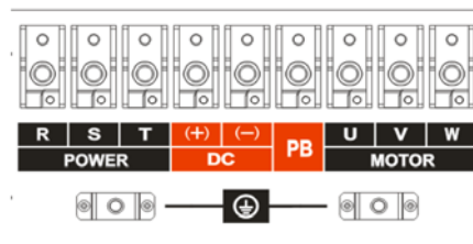
Рис. 3-14. Схема силовых клемм ПЧ мощностью 45~90 кВт
