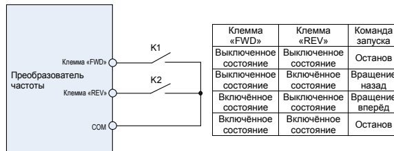
Рисунок 6-8. Настройки режима двухпроводного управления 1
