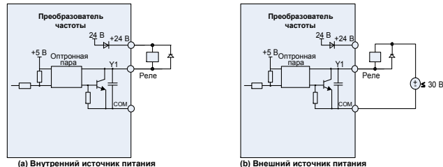
Рис. 3-21. Схема подключения выходных клемм с использованием реле
