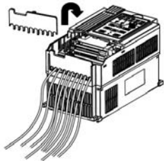
Рис. 3-7(g). Демонтаж и монтаж проводоразделительной пластины
